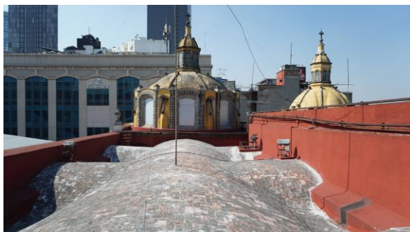
Figura 1. Estado Inicial de extradós de bóveda de Nave Principal.
